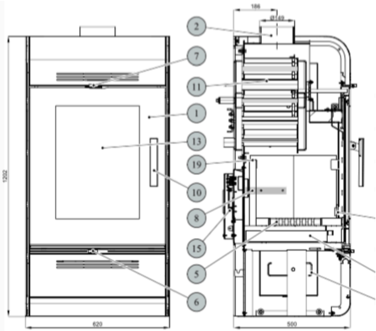
Informativní rozměr topeniště
